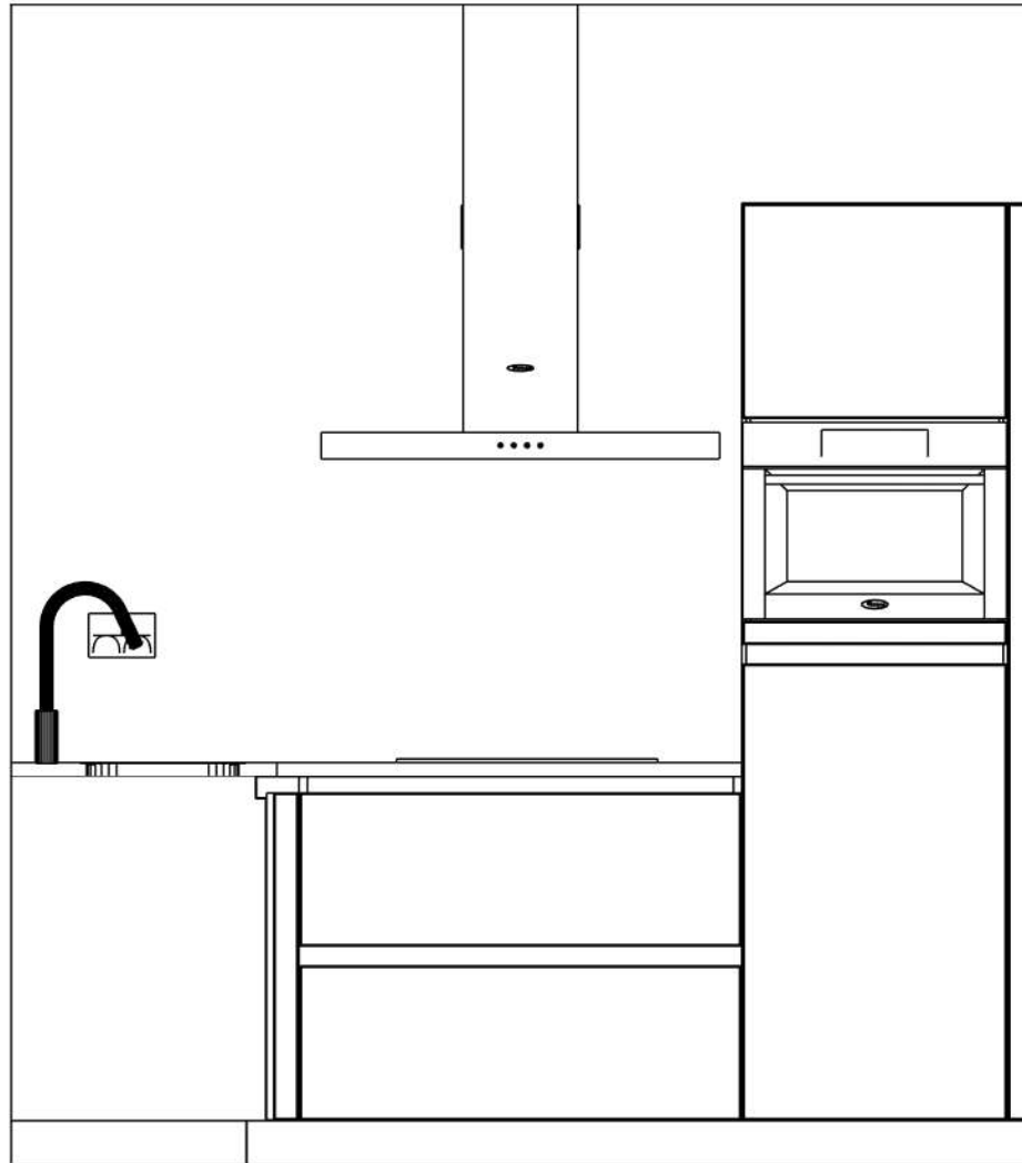
Vooraanzicht wand 2
